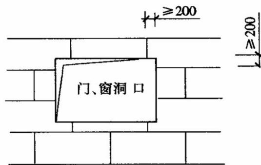
图 6.1.9 (b) 门窗洞口 EPS 板排列
