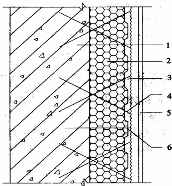
图 6.4.1 有网现浇系统
