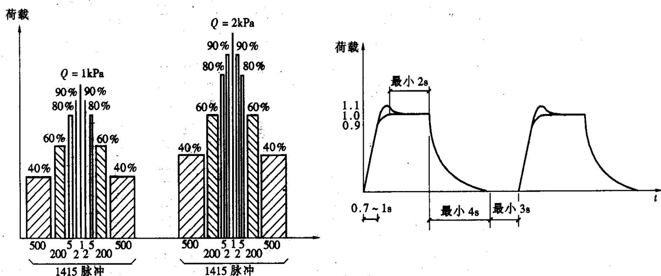
图 A.3.3 加压步骤及压力脉冲图形
