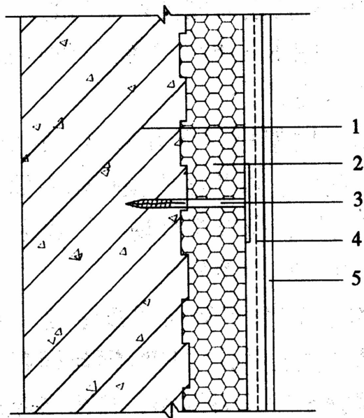
图 6.3.1 无网现浇系统
