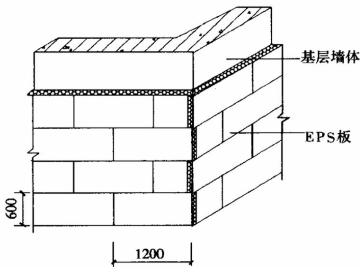
图 6.1.9 (a) EPS 板排板图
