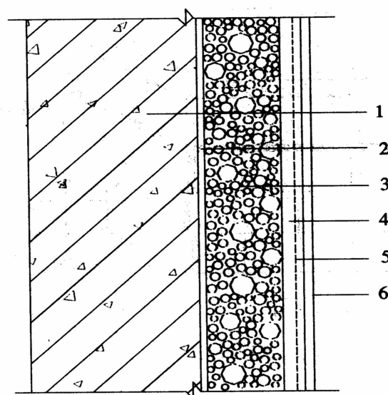
图 6.2.1 保温浆料系统
