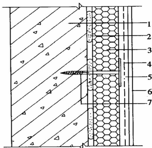
图 6.1.1 EPS 板薄抹灰系统
