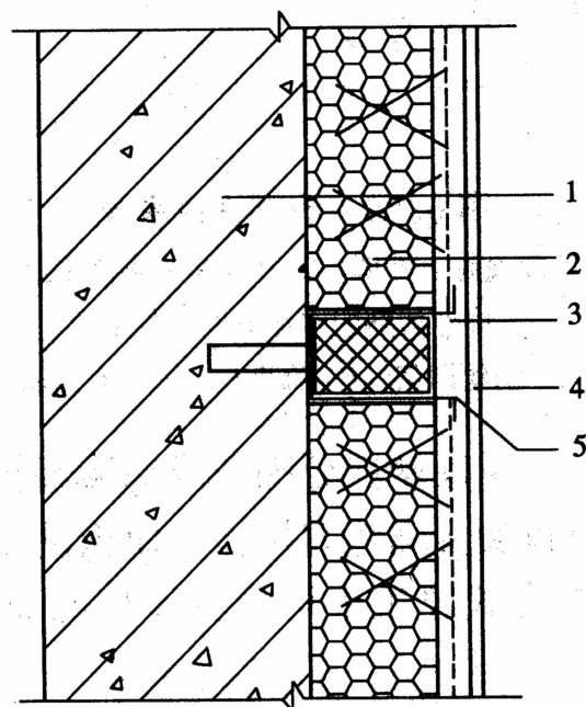
图 6.5.1 机械固定系统
