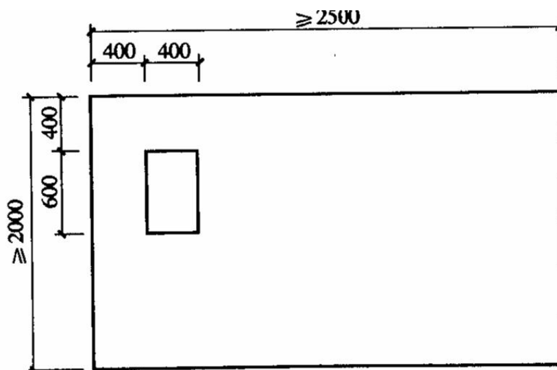
图 A.2.1 试样
