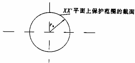
图 B.0.1-2 单支避雷针的保护范围 ( h > h_r )
